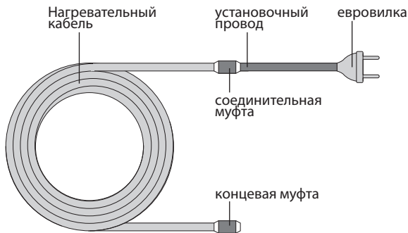
Рис. 1. Конструкция секции нагревательной AURA FS
